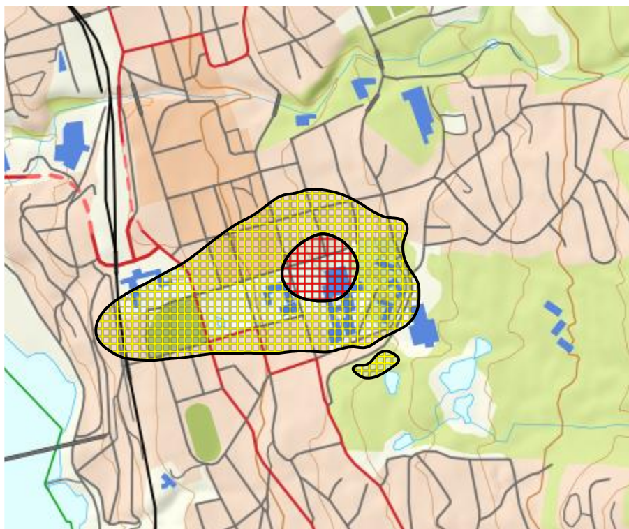
Figur 8-1. Støysonekart etter T-1442/2021 for landingsplassen. M 1:15 000.
