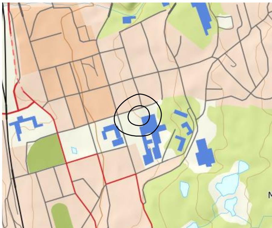
Figur 8-2. Kartleggings- og tiltaksgrenser i henhold til forurensingsforskriften. Kotene viser L_{Aeq} 58 og 65 dBA. M 1:10 000.
